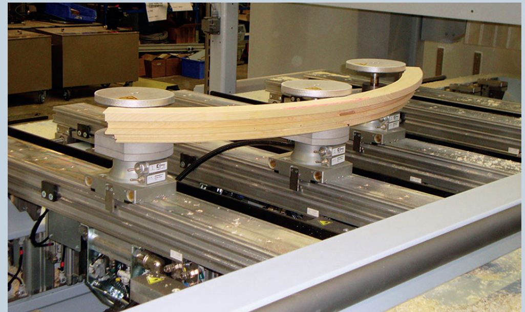
Produktion von Spezialfenstern auf dem CNC-gesteuerten Bearbeitungszentrum
